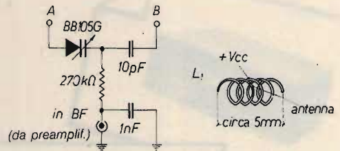
Modulatore per generatore VHF.
