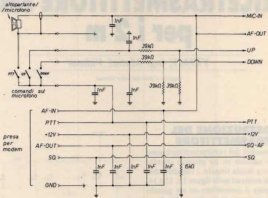
figura 11 RTX FM per i 2 m, connessioni varie.
