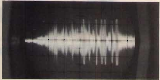
Agendo sul compensatore C_{V3} è possibile estendere o ridurre l'ampiezza della banda esplorata.
