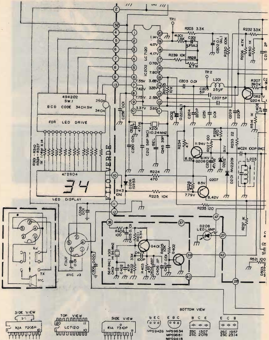
Schema elettrico della versione INTEK. Si vede bene il filo verde da togliere per la modifica
