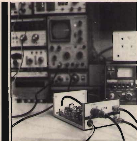
foto 2 Per tarare adeguatamente il "LYNX", è necessario poter disporre di un oscilloscopio e di un generatore.
