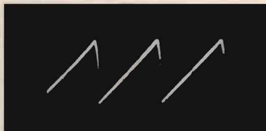
foto 7 Forma d'onda rilevata ai capi del trimmer P_3 .
